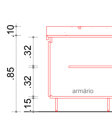
CORTE B - BANCADA 5 ESCALA: 1/25
