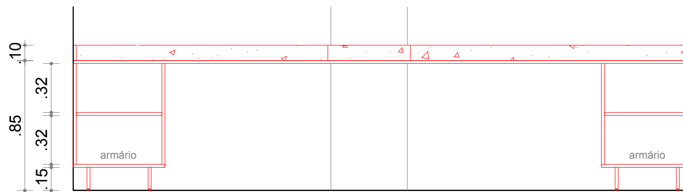
CORTE A - BANCADA 5 ESCALA: 1/25
