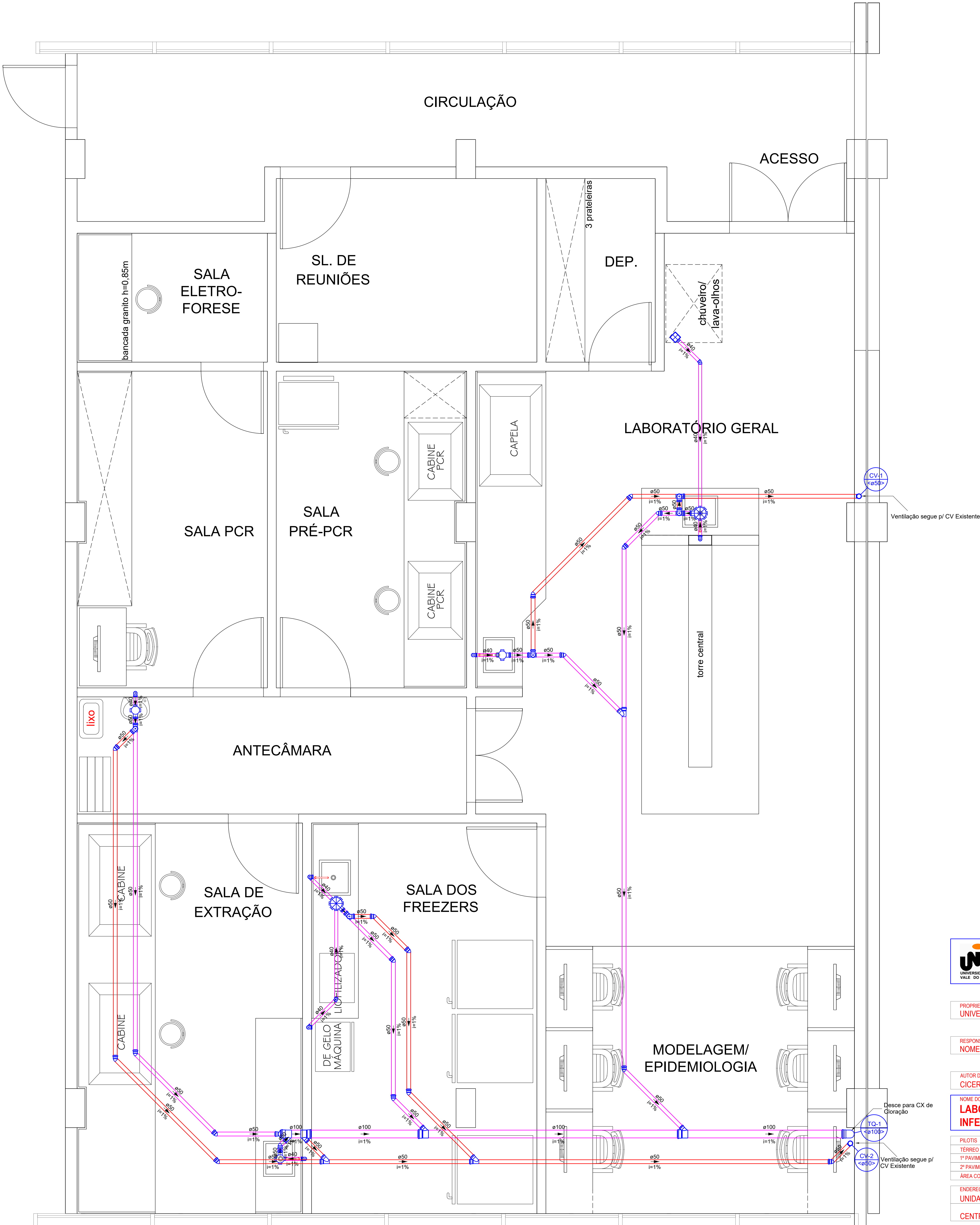
Planta Sanitária Escala 1:25
